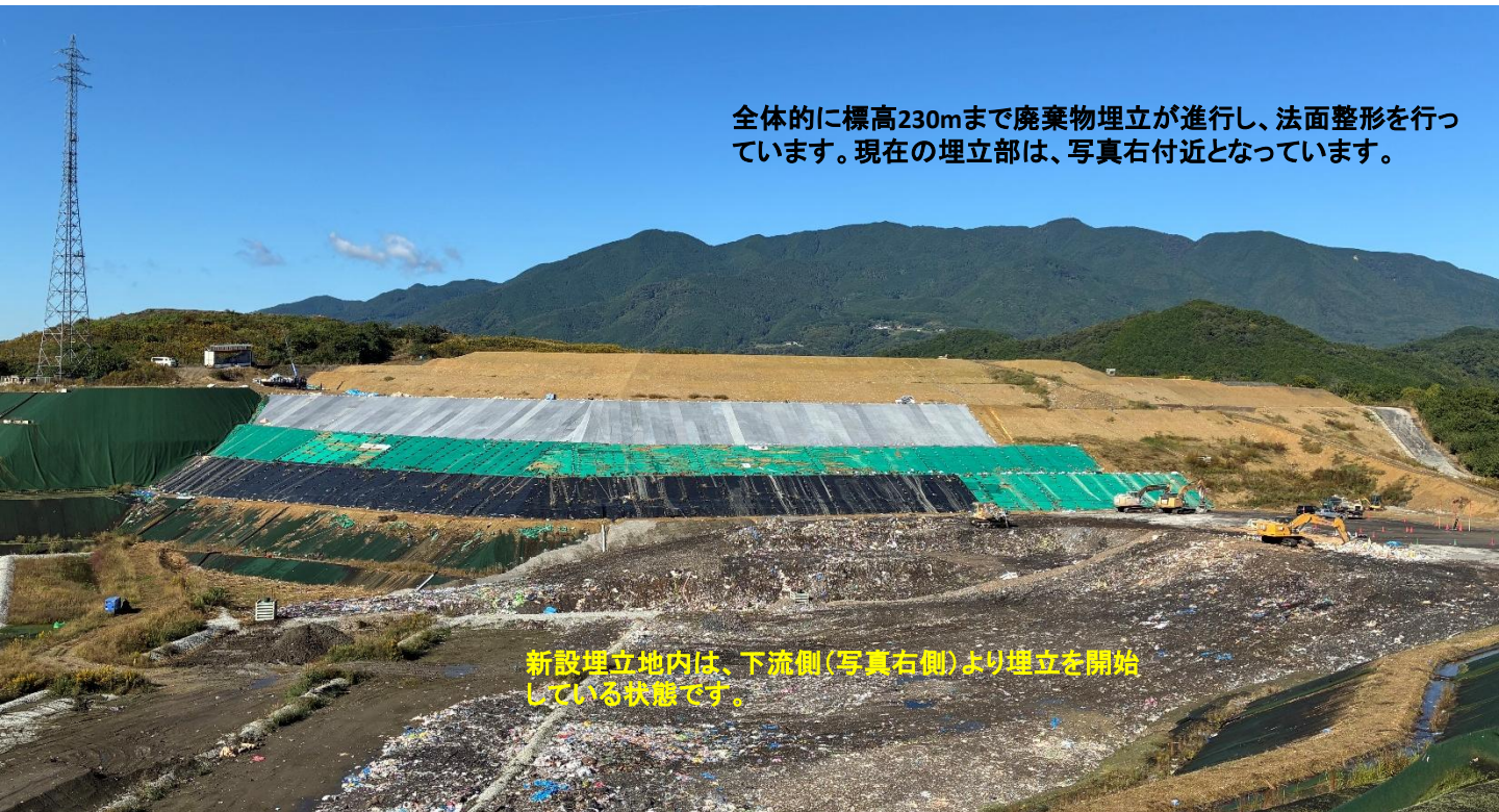
写真① 現在の廃棄物埋立部と新設埋立地北側(下流側)の状況
